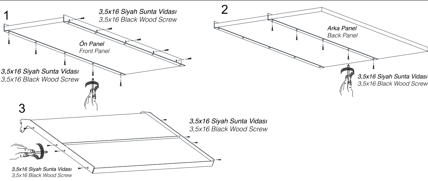
3,5x16 Siyah Sunta Vidası 3,5x16 Black Wood Screw
