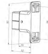
Ayarlanabilir Plastik Bağlantı Adjustable Connector
