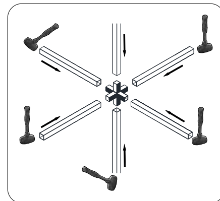
Altı Yönlü Plastik Bağlantı / Six Way Plastic Connection
