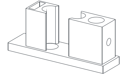
Konnektör Connector 2 Adet / 2 Pcs.
