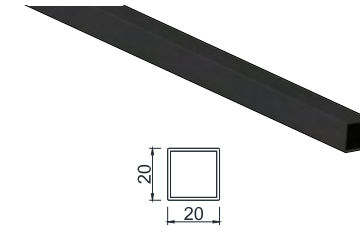
Puzzle Tımsız Alüminyum Profil / Puzzle Aluminium Profile without Nail
