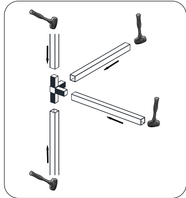
Dört Yönlü Köşe Plastik Bağlantı / Four Way Corner Plastic Connection
