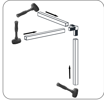
Üç Yönlü Köşe Plastik Bağlantı / Three Way Corner Plastic Connection
