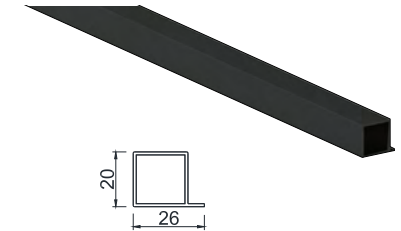
Puzzle Tımsız Alüminyum Profil / Puzzle Aluminium Profile with Nail
