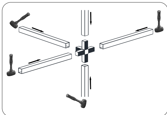
Beş Yönlü Plastik Bağlantı / Five Way Plastic Connection
